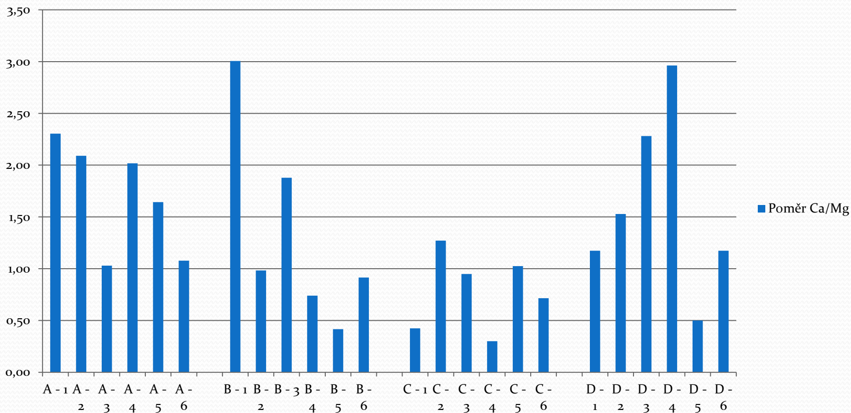
Poměr průměrných hmotnostních koncentrací Ca/Mg
